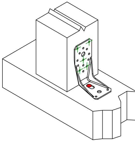
Montering med 1 beslag
