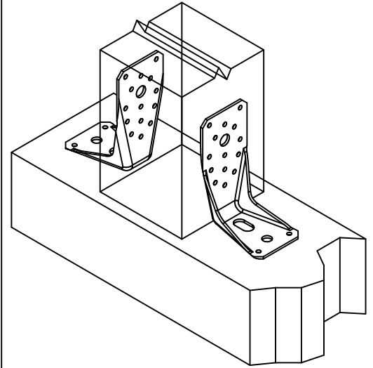
Montering med 2 beslag
